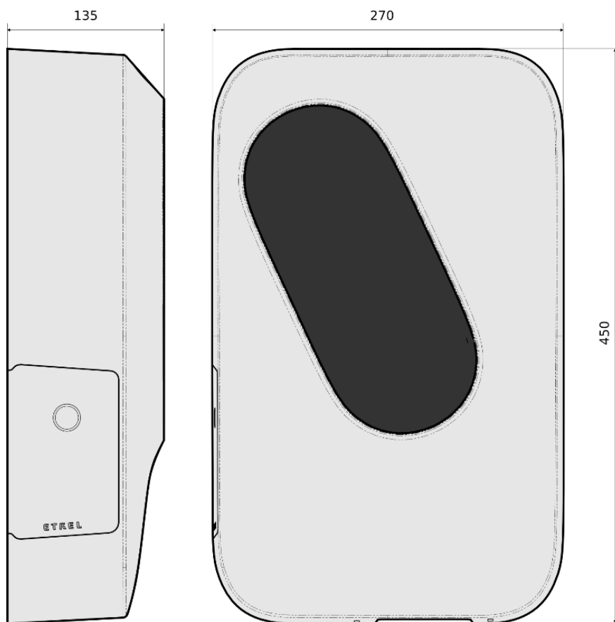
Afbeelding 4: Afmetingen van het INCH laadstation
